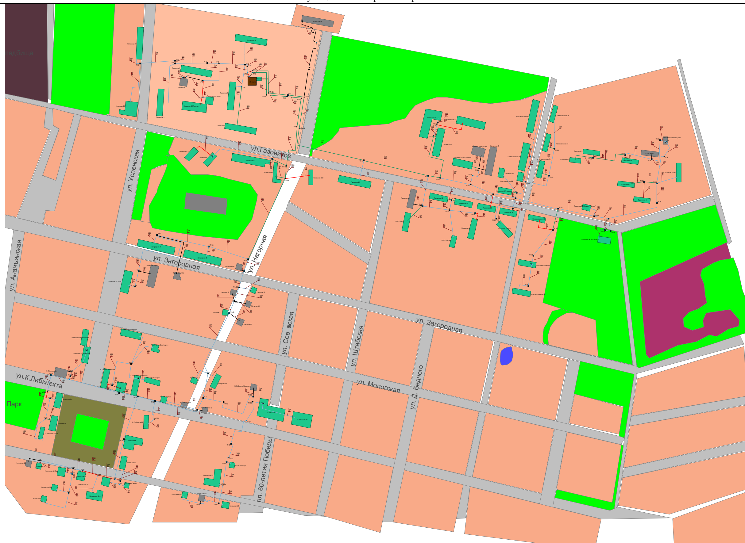
Рис. 4 Схема тепловых сетей котельной «26 квартал» в режиме наладки
