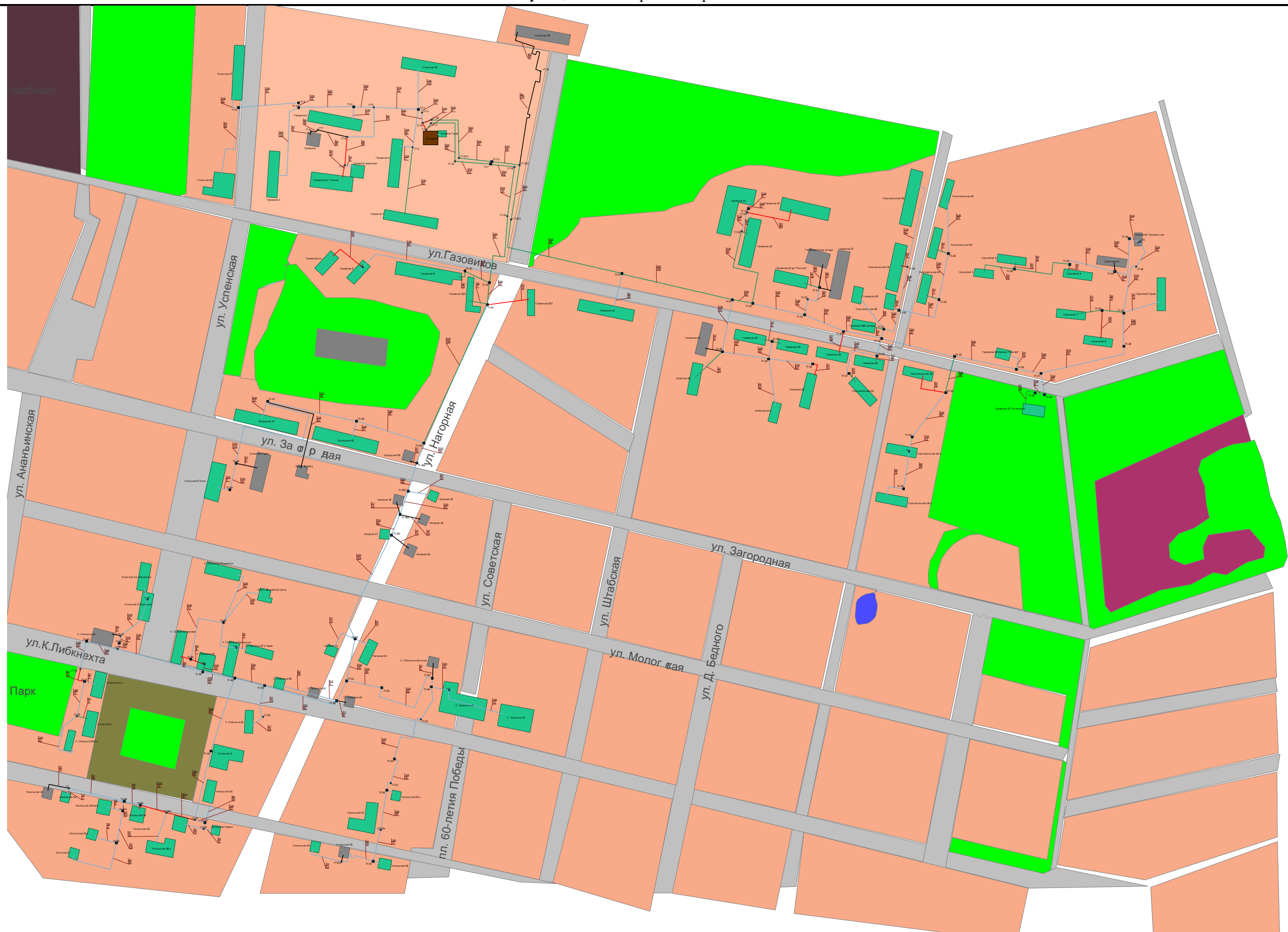
Рис.8 Котельная «26 квартал» – наладочный режим системы теплоснабжения
